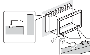
1 Накладная рамка
