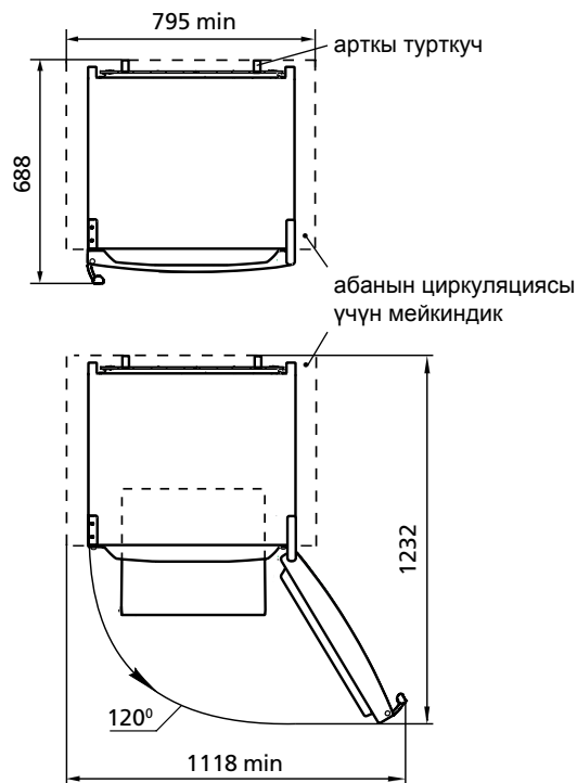
2-сүрөт – Муздаткыч (үстүнөн)
