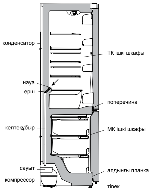
Сурет 6 — TK еріген суды ағызу схемасы
