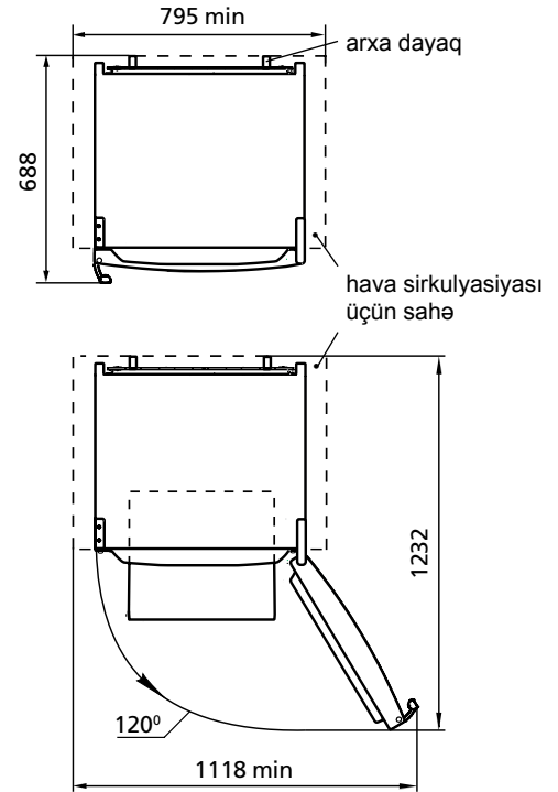
Şəkil 2 — Soyuducu (yuxarıdan görünüşü)
