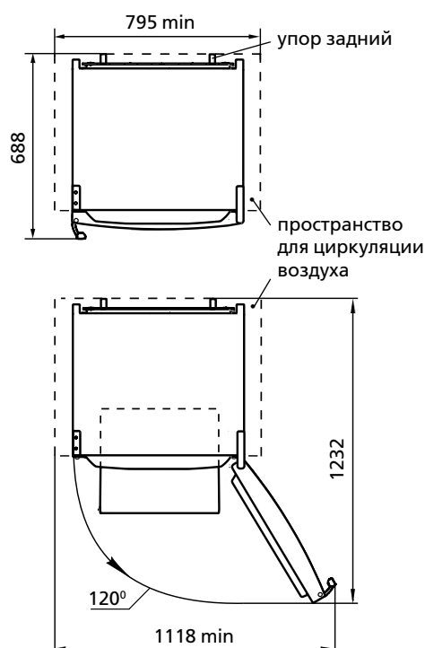
Рисунок 2 — Холодильник (вид сверху)
