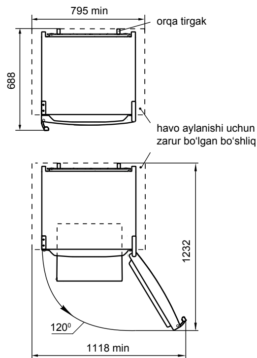
2-расм — Совутгич (тепадан кўриниши)
