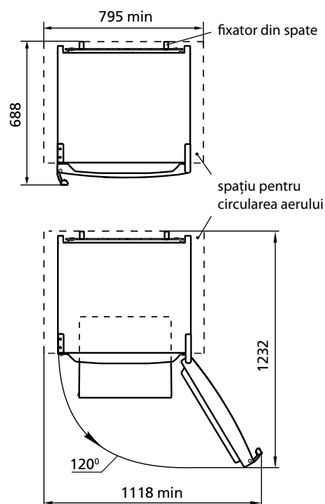
Figura 2 – Frigider (privire de sus)
