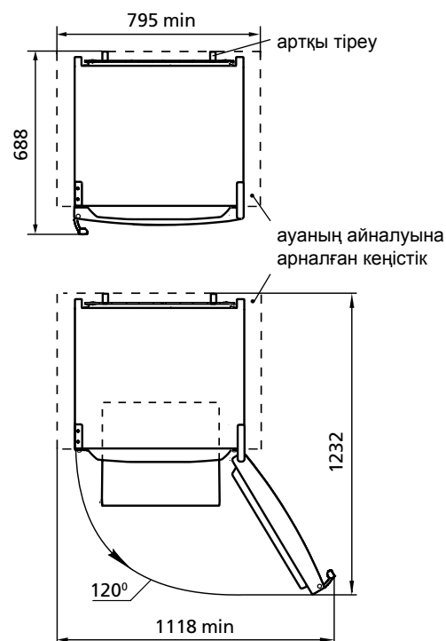
Сурет 2 — Тоңазытқыш (үстінен қарағанда)
